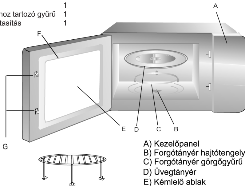
Grillező állvány (csak a grillező modellekhez)
